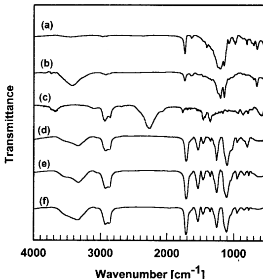
Fig. 2. FT-IR spectra ((a) FA, (b) FA/TG macromonomer, (c) HMDI, polyurethane with Z-DOL content (d) 10 wt %, (e) 1 wt %, (f) 0 wt %).
